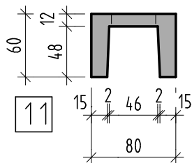
QUERSCHNITT
