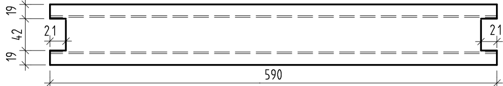
QUERSCHNITT
